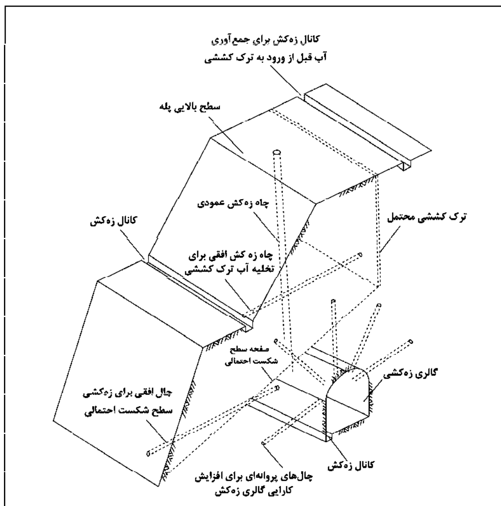
شکل ۷-۲- نمایش روش‌های مختلف زه‌کشی در معادن روباز
