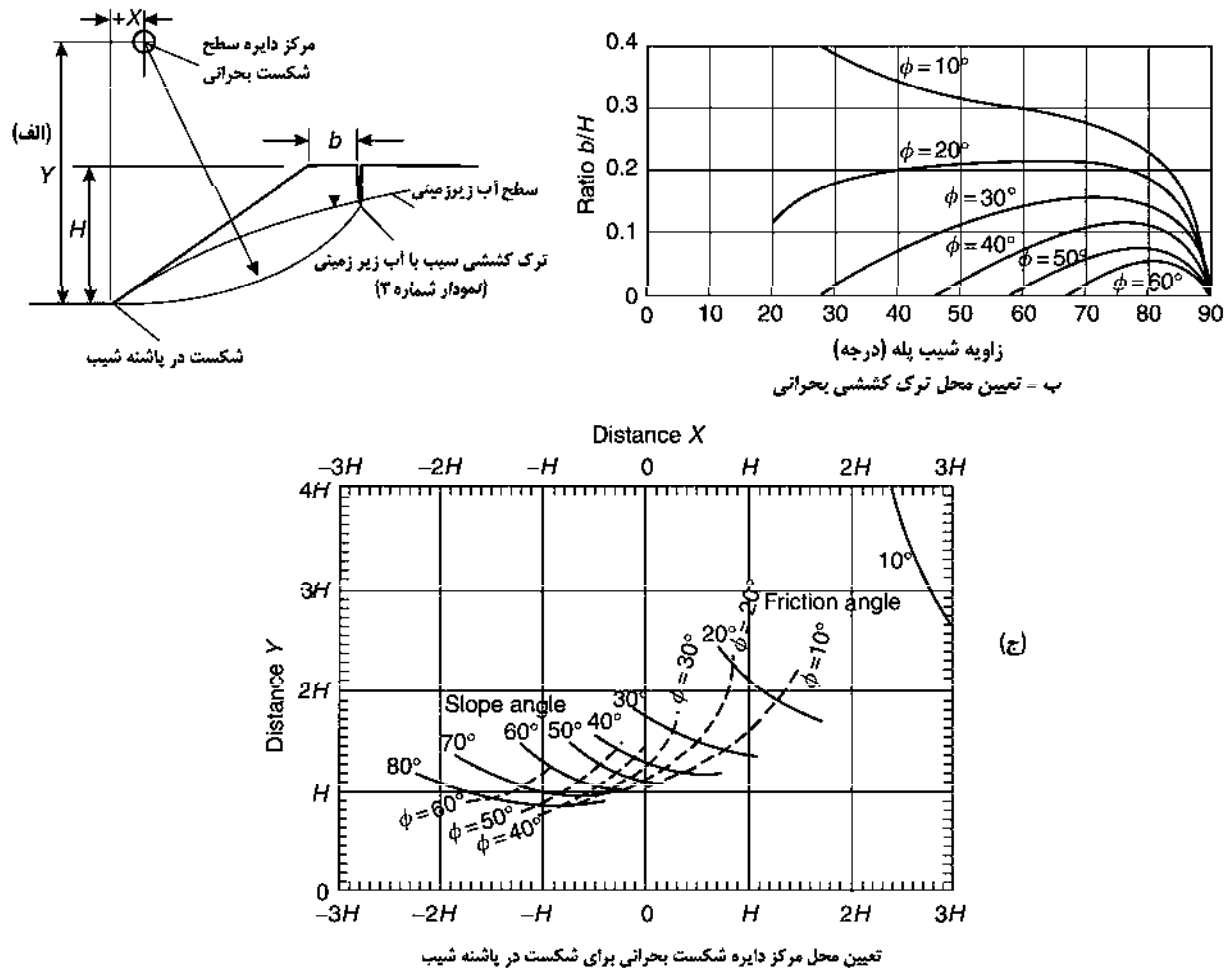
شکل ۹-۵- محل سطح لغزش بحرانی و ترک کششی بحرانی برای یک شیب با فشار آب زیرزمینی
