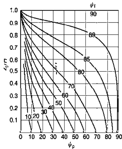
شکل ۵-۱۶- موقعیت ترک کششی بحرانی برای یک پله خشک، (الف) عمق ترک کششی (ب) موقعیت ترک کششی بحرانی پشت پیشانی پله.
