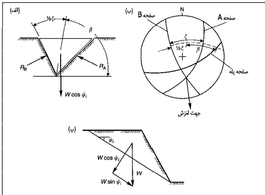
شکل ۵-۲۱- بردار نیروهای وارد بر گوه و تعیین زاویه‌های مربوط به آن‌ها
