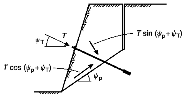
شکل ۵-۱۷- تقویت شیب با استفاده از پیچ‌سنگ کششی
