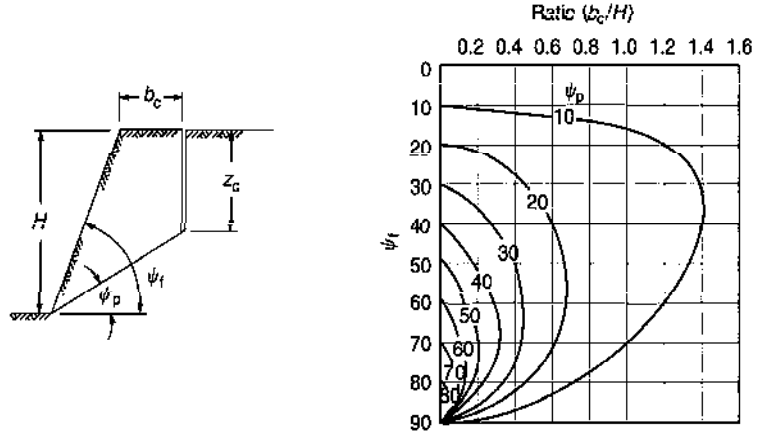
شکل ۵-۱۶- موقعیت ترک کششی بحرانی برای یک پله خشک، (الف) عمق ترک کششی (ب) موقعیت ترک کششی بحرانی پشت پیشانی پله.
