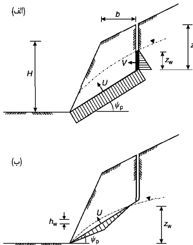
شکل ۵-۱۵- حالت‌های ممکن فشار آب زیرزمینی در شکست صفحه‌ای، (الف): فشار یکنواخت روی سطح لغزش در صورت بسته شدن مسیر زهکشی در پاشنه شیب (ب): فشار مثلثی روی سطح لغزش در شرایطی که سطح آب زیرزمینی زیر قاعده ترک کششی واقع است.
