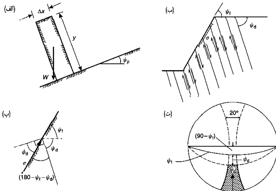
شکل ۵-۲۹- شرایط سینماتیکی برای لغزش خمشی قبل از واژگونی (الف): نسبت ارتفاع به پهنای بلوک برای واژگونی (ب): جهت‌های تنش و جهت‌های لغزش در شیب سنگی (پ): شرایط لغزش بین لایه‌ای (ت): بررسی سینماتیکی به وسیله تصاویر استریوگرافیک.
